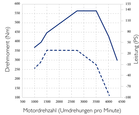
FIA e-VGT 156 PS Drehmoment/PS
