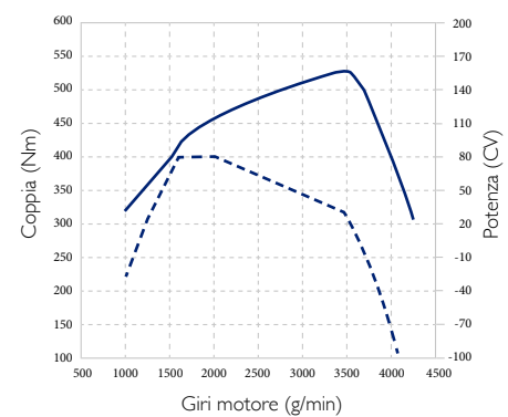
FIA e-VGT 160 CV Curve di coppia e potenza
