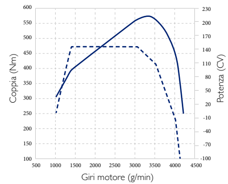
FICWG 140 CV Curve di coppia e potenza
