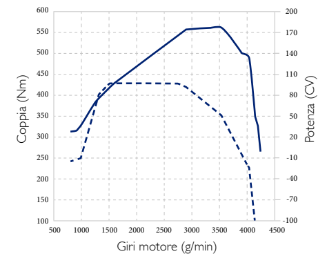
FIA e-VGT 140 CV Curve di coppia e potenza
